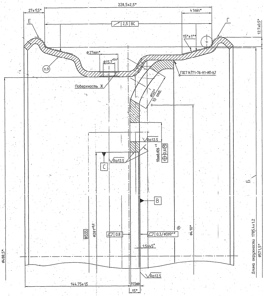
Рисунок - Колесо 9,00x22,5
