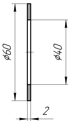
Рисунок - Шайба типа 54321-3501160
