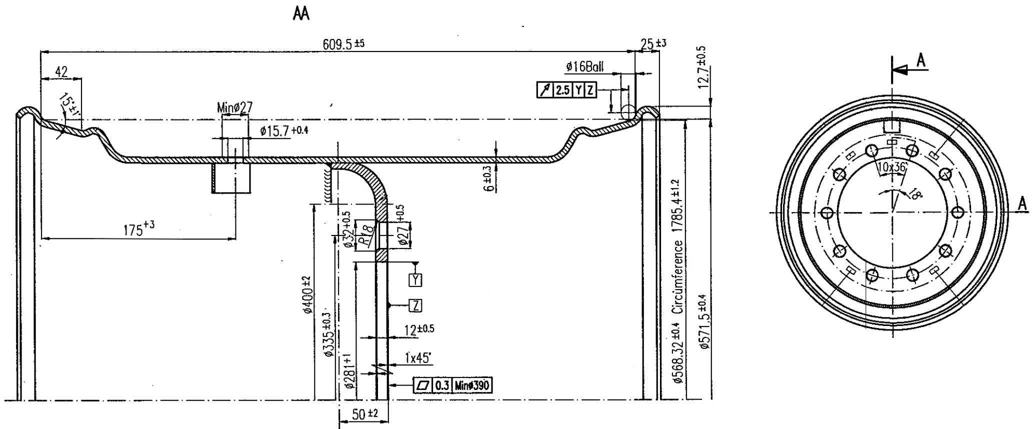
Рисунок - Диск колесный 24x22.5
