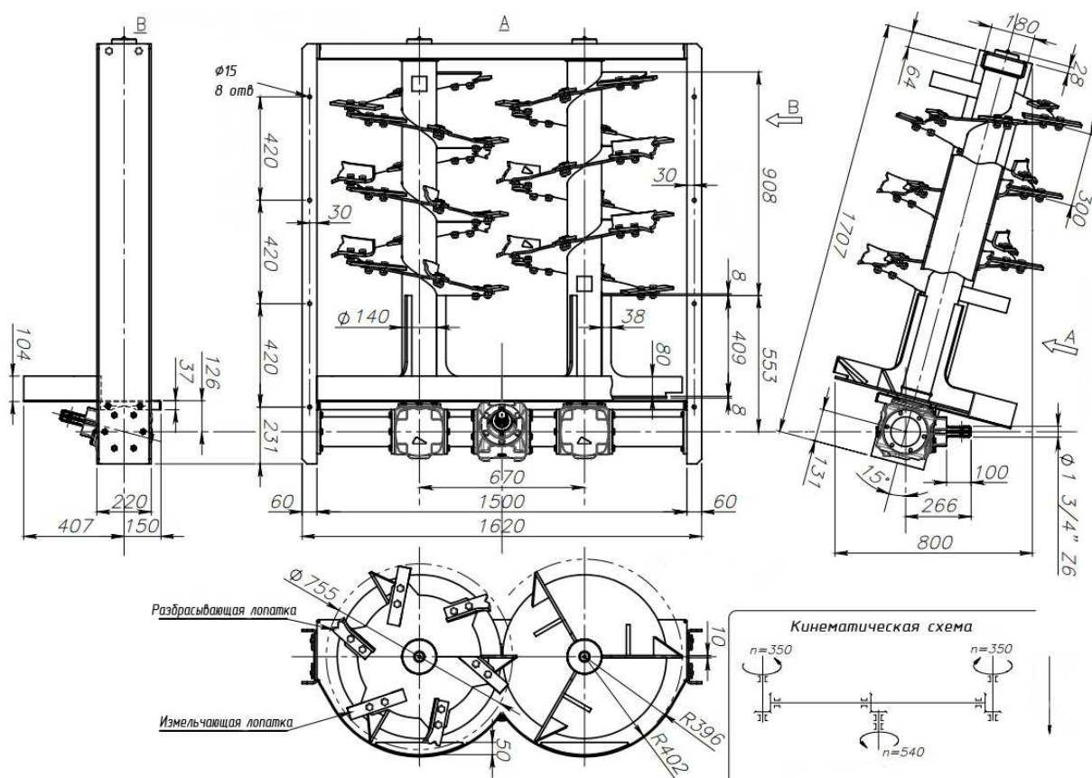
Рисунок – Устройство разбрасывающее для машин внесения твердых органических удобрений типа МТТ-9-1
