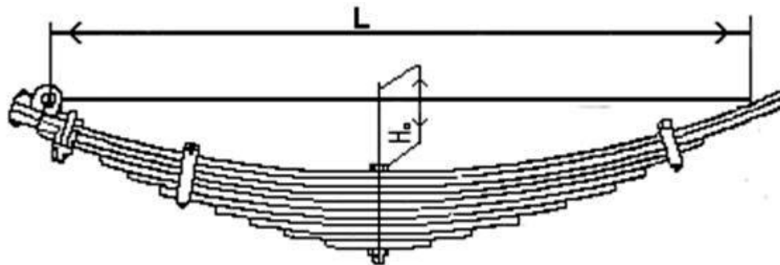
Рисунок - Рессора типа 5232В-2912012-02 задняя или ее аналог
