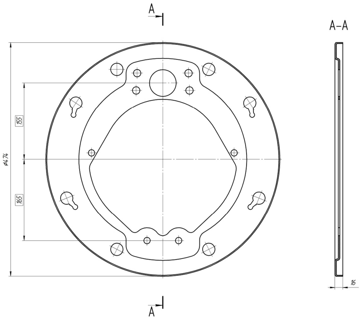
Рисунок - Общий вид щита тормоза типа 5336-3501150
