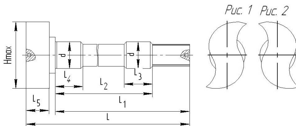
Рисунок - Кулак разжимной типа 54326-3502110/111 для тормозной системы
