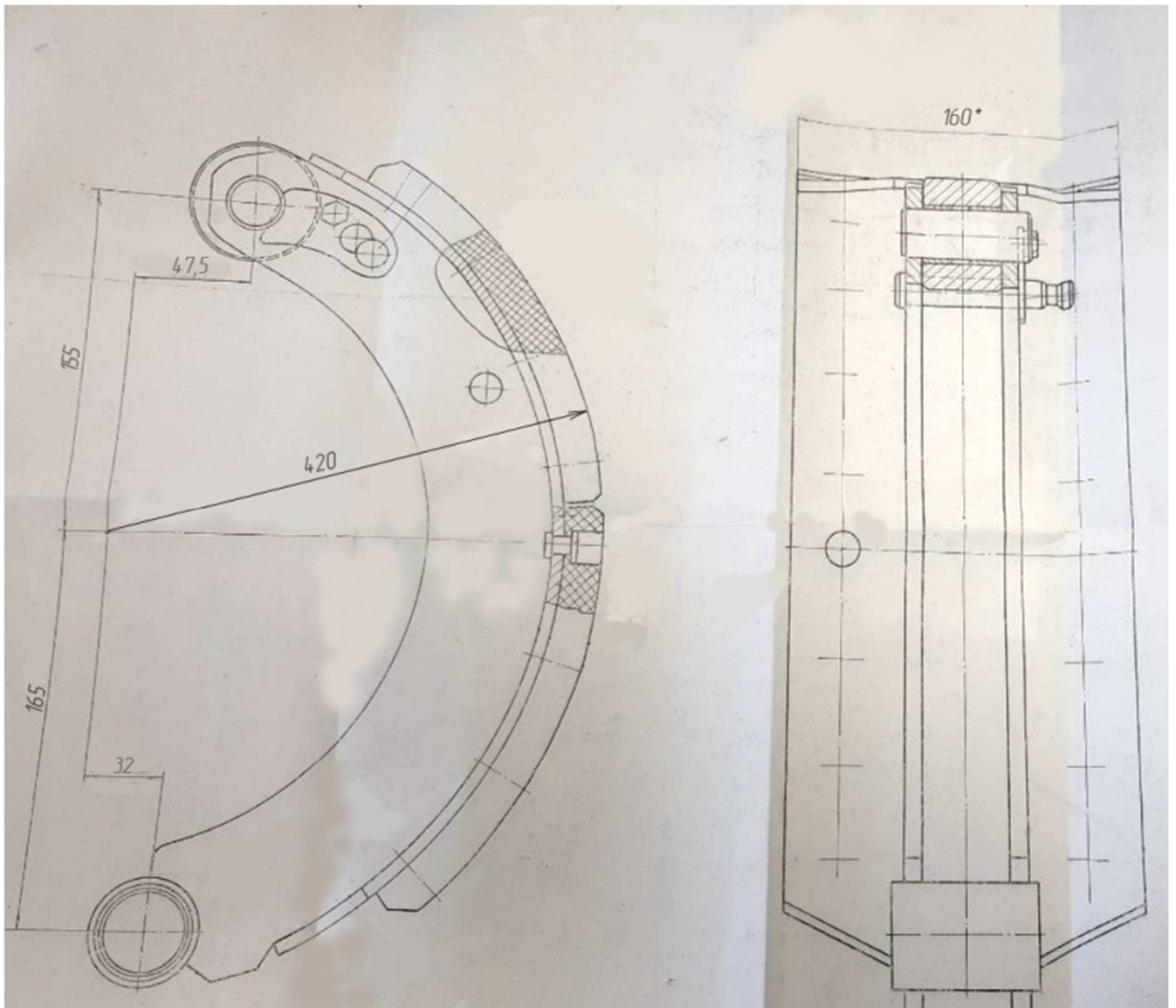
Рисунок - Общий вид колодок тормозных типа 63171-3501090/091
